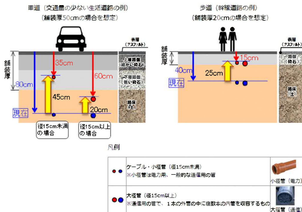
※舗装厚は、当該道路の交通状況、地盤状況に応じて設定される 図-8 「電線等の埋設物に関する設置基準」の見直しイメージ図（出典：国土交通省HP）
